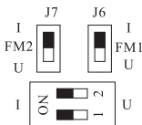
Переключатели и клеммы платы управления преобразователя частоты серии FCI
